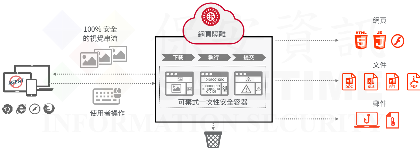
圖一：賽門鐵克網頁隔離的流程圖
