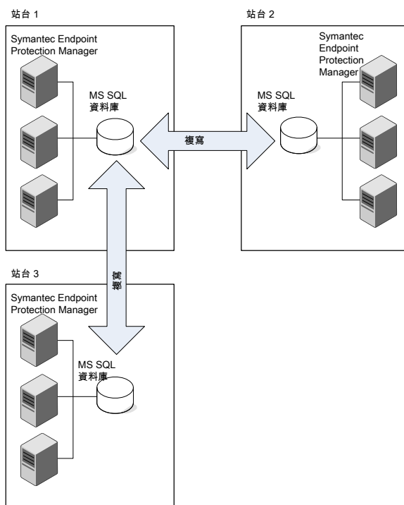
圖 35-1 主站台與兩個遠端站台之間進行複寫的方式
