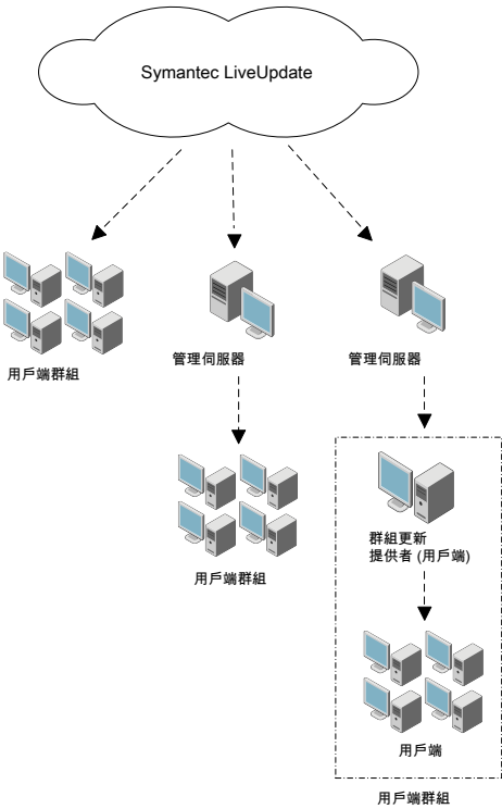
圖 8-1 較小型網路的派送架構範例
